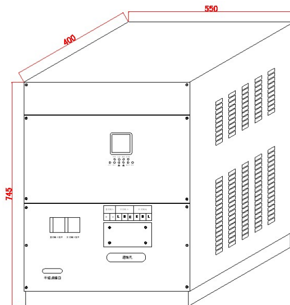
5KVA-10KVA 单相工频电力 UPS 外形机械尺寸图
